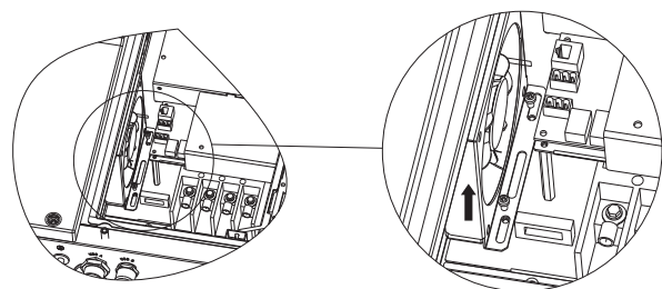
Fig 9.2 Vista do ventilador interno
